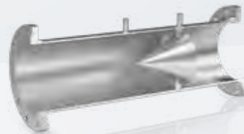
OPTIBAR MR 6300 Débitmètre à cône avec robinets simples
