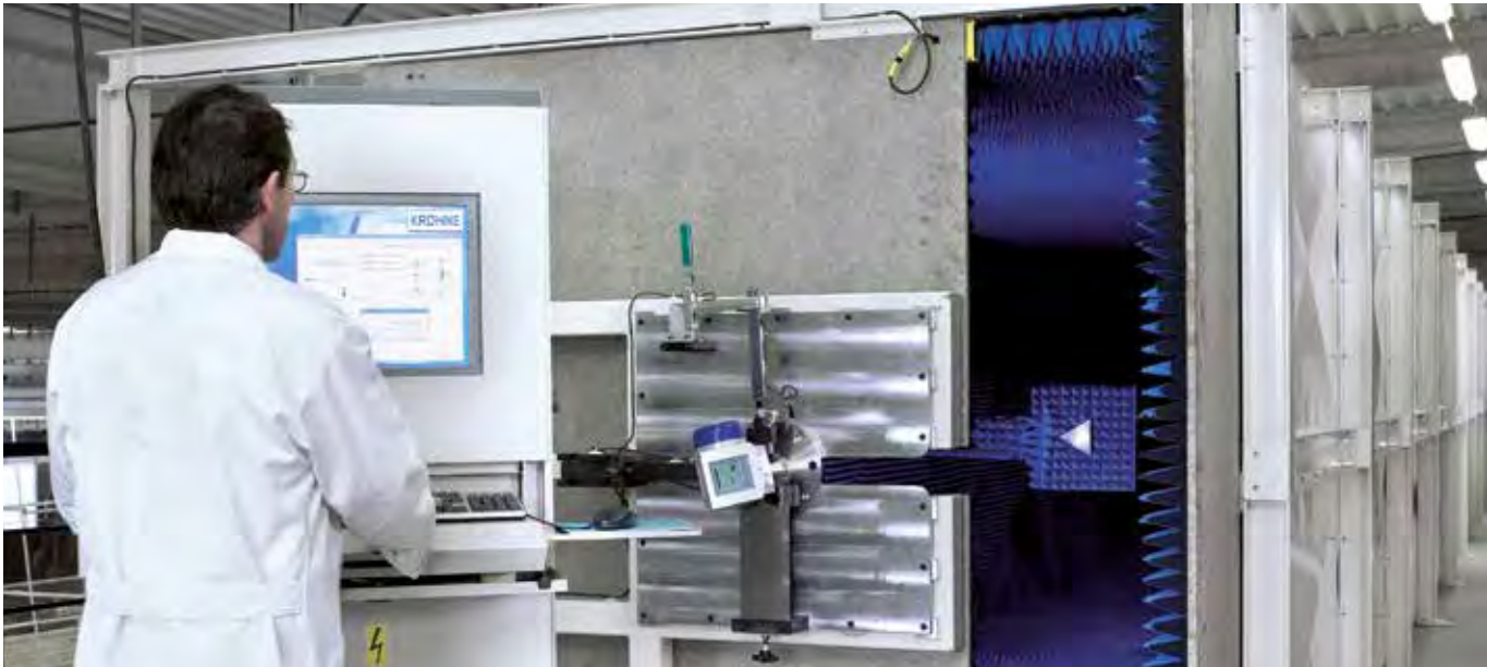
Section d'étalonnage pour transmetteurs de niveau FMCW
